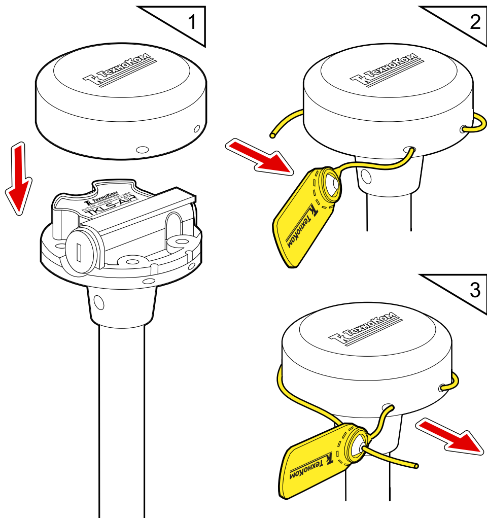
Рис.25. Пломбировка корпуса датчика
