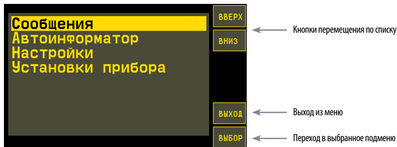
Рис. 19. Главное меню.
