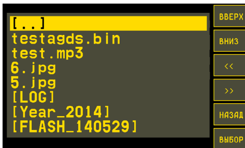
Рис.86. Содержимое SD-карты.
