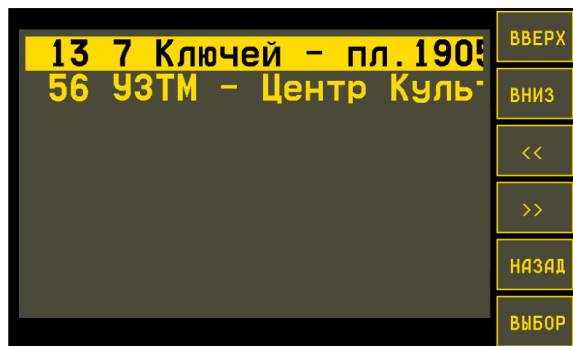
Рис.71. Выбор маршрута.
