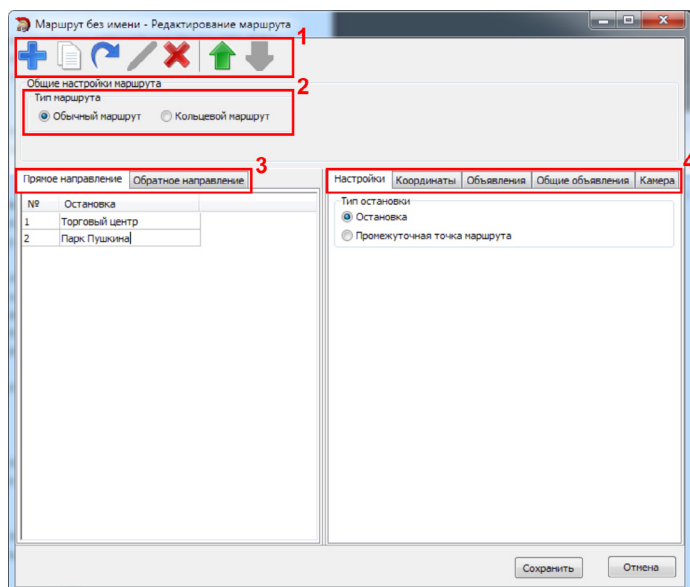
Рис.59. Редактор маршрута.
