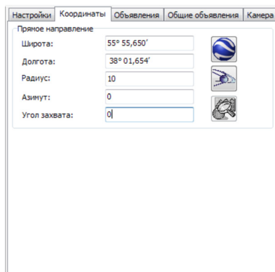
Рис.61. Вкладка «Координаты».
