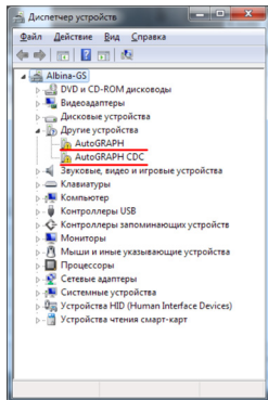
Рис.98. Новые устройства.
