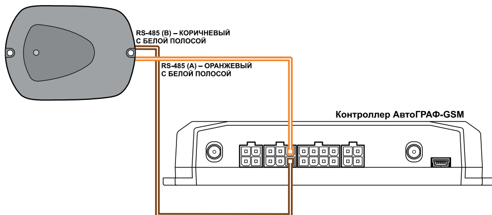
Рис.14. Схема соединения бортового контроллера и TKFC Plus
