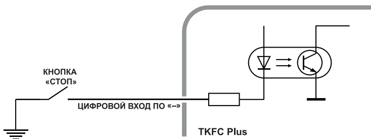
Рис.8. Внутренняя схема подключения дискретного входа 3
