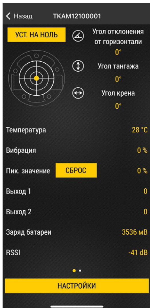
Рис.32. Установка на ноль.
