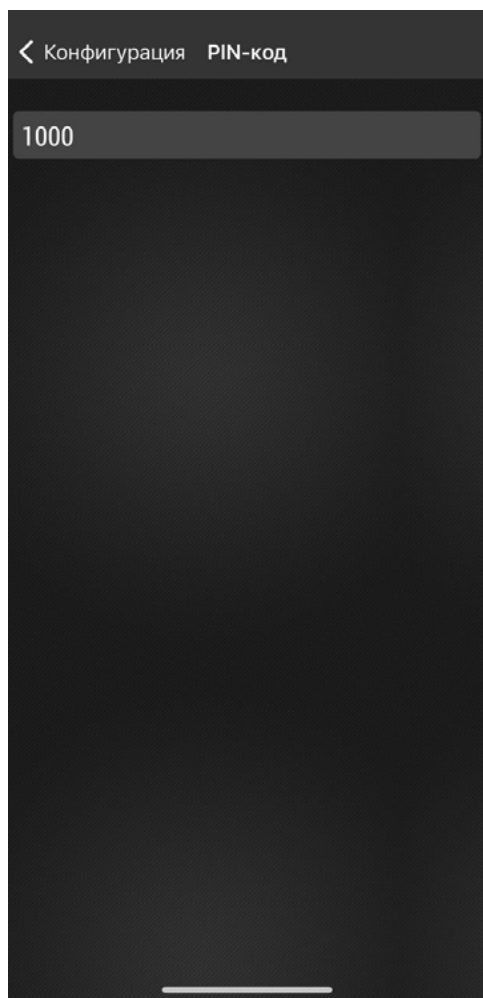
Рис.29. Ввод PIN-кода.
