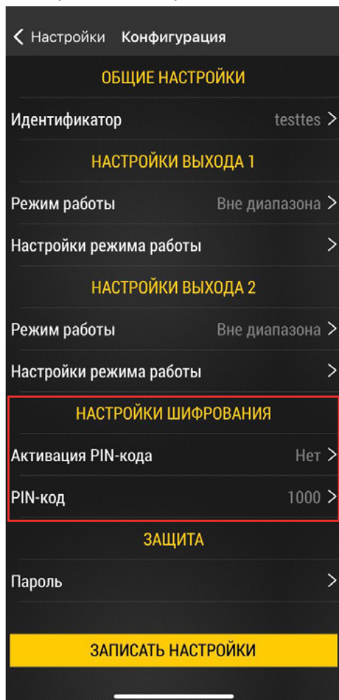
Рис.27. Настройки шифрования.
