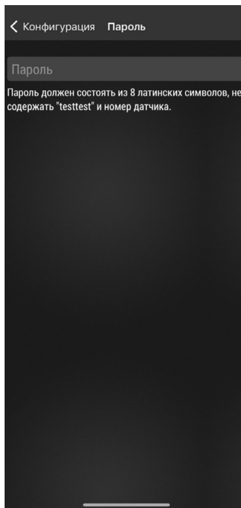
Рис.30. Ввод Пароля.
