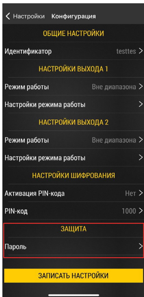
Рис.31. Настройки защиты.
