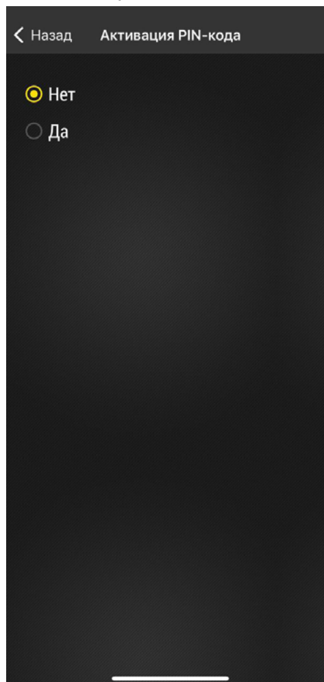
Рис.28. Активация PIN-кода.
