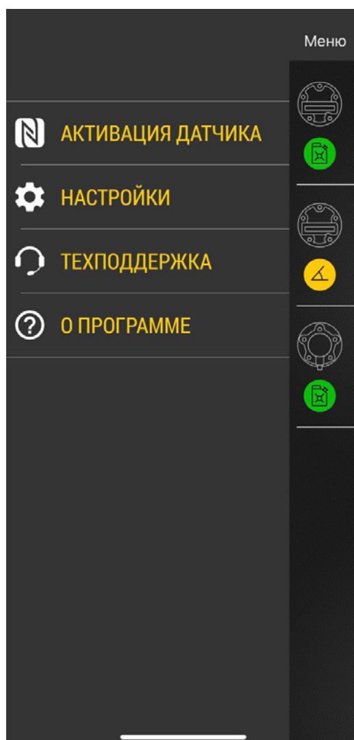
Рис.34. Активация датчика.
