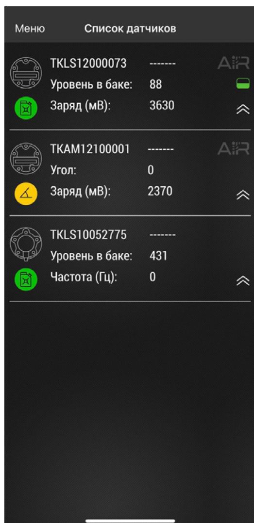
Рис.33. Найденные датчики.
