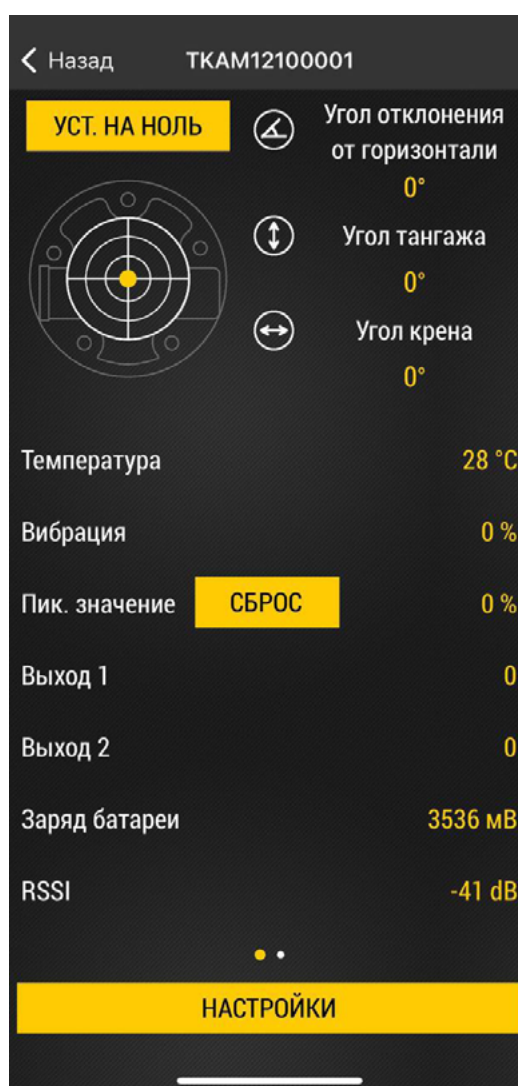
Рис.10. Рабочий экран.
