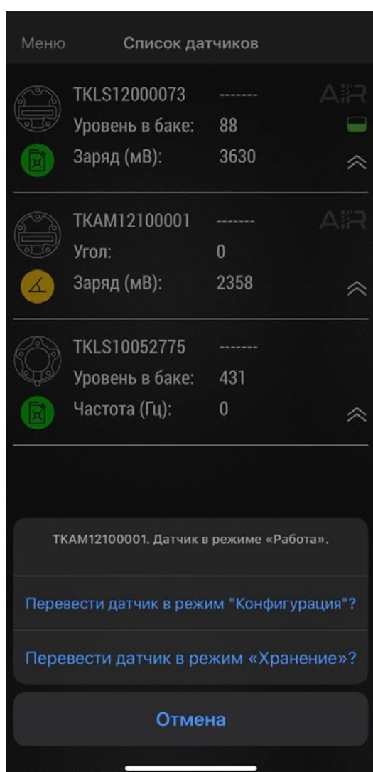
Рис.9. Выбор режима.
