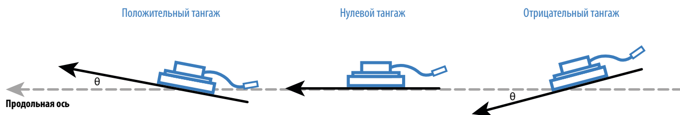
Рис.26. Измерение угла наклона относительно продольной оси датчика.
